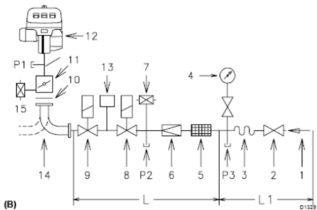
Godkända gasarmaturset i fig. EN 676 standard
