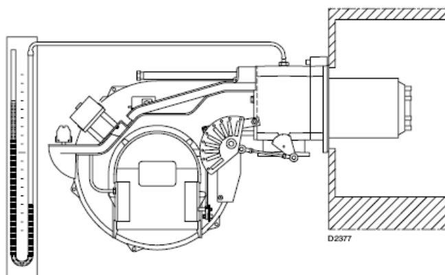
(D) Servomotor
