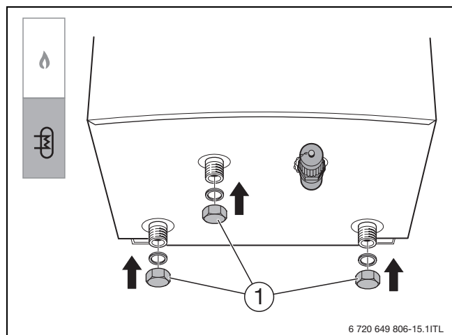
Fig. 11 Montering af blindpropper
